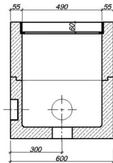
przekrój poprzeczny
